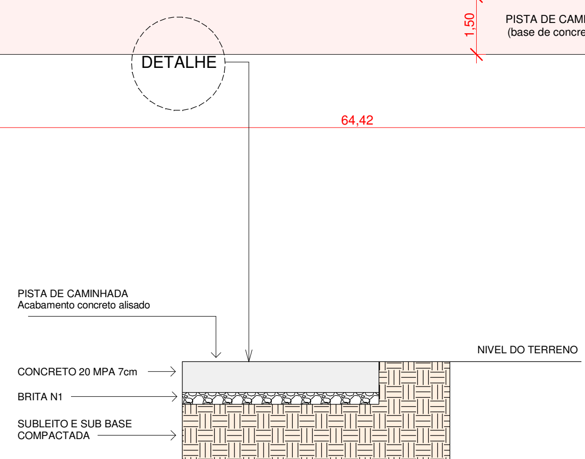
2 DETALHE PISO PISTA CAMINHADA 1 : 10
